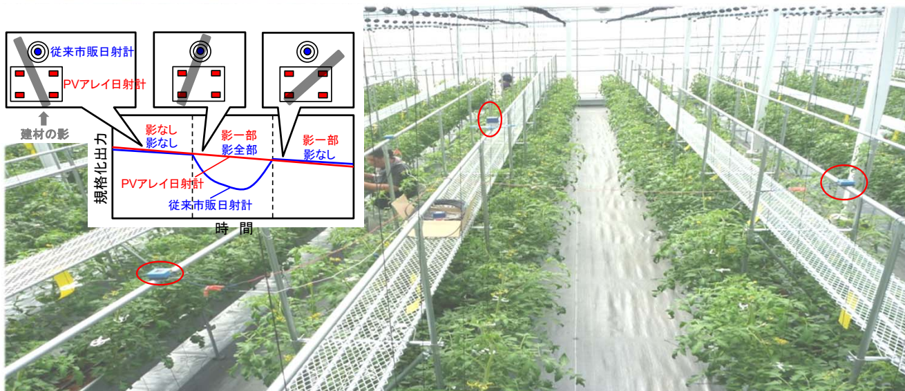
【ビニールハウス内で複数接続(アレイ接続)している様子です】 ※○部分がPVSS-03です
