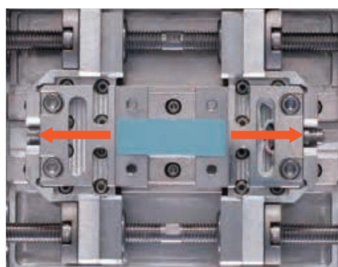
【引張試験時の観察点の視野ドリフト例】
